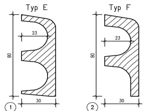
Heizrohrabdeckleiste
