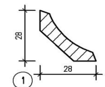
Hohlkehlleiste
