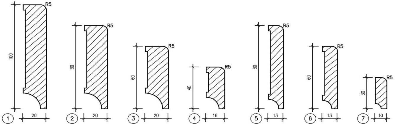
Fußleiste 10 - abgerundet R=5mm
