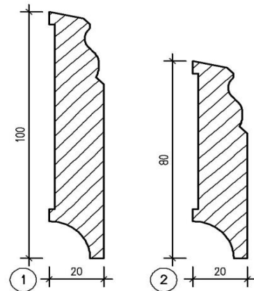
Berlinerprofil 30
