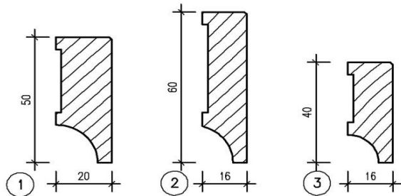
Fußleiste 20 - scharfkantig 1mm
