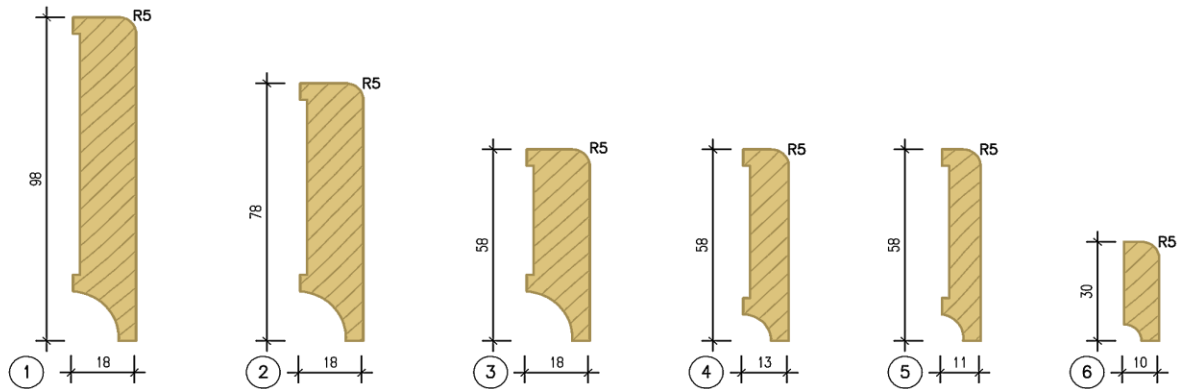
Fußleiste 10 - abgerundet R=5mm
