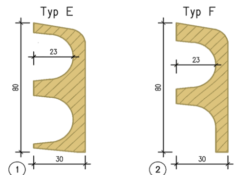
Heizrohrabdeckleiste 80
