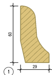
Sockelleiste 40
