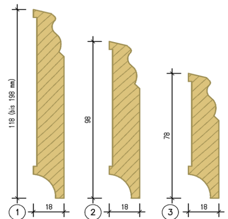
Berlinerprofil 30
