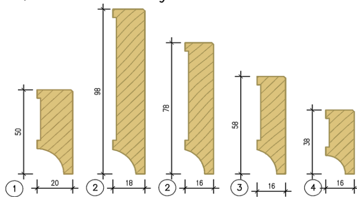
Fußleiste 20 - scharfkantig 1mm
